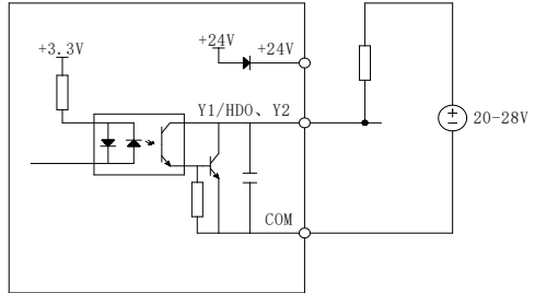
图 2-14 使用外部电源
