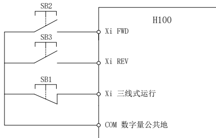
图 5-12 三线式模式示意图
