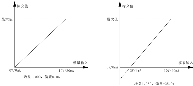
图 5-18 AI 增益和偏置设置示意图
