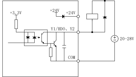
图 2-16 使用外部电源
