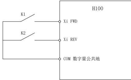
图 5-11 两线式模式示意图
