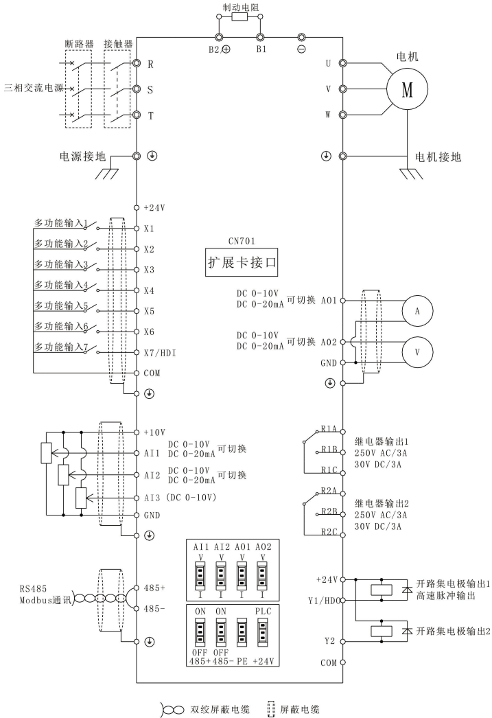
图 2-4 标准接线图
