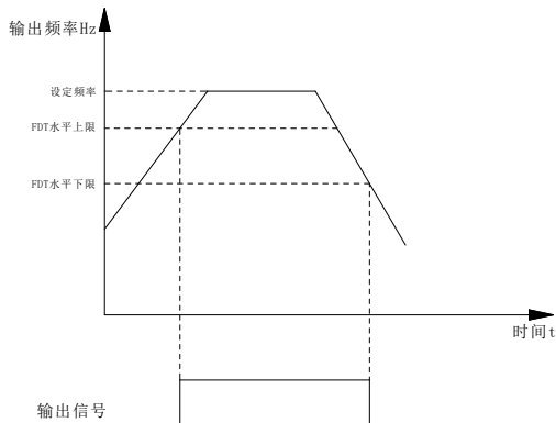
图 5-13 FDT 工作示意图
