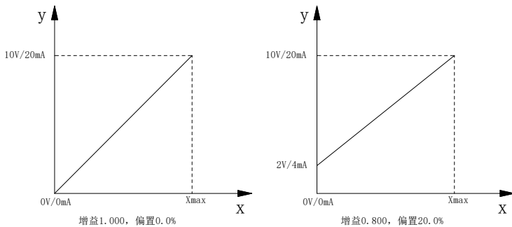
图 5-19 AO 输出示意图
