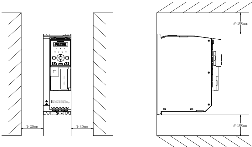
图 2-2 H100-4T15GB 及以下功率等级安装方向和空间要求
