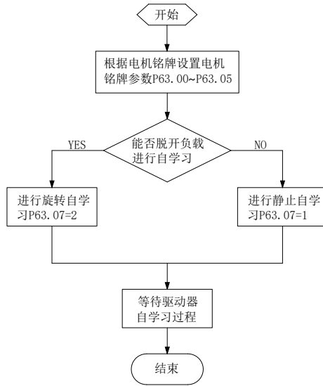
图 3-3 电机自学习流程
