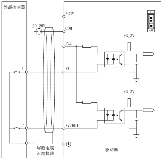
图 2-8 使用外部电源干接点方式
