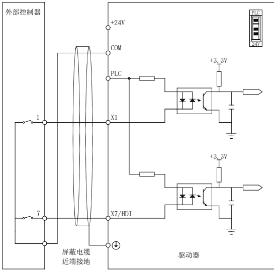
图 2-7 使用内部电源干接点方式
