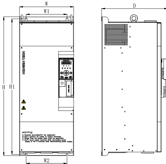
图 8-3 H100-4T18.5G~H100-4T30G 安装尺寸示意图
