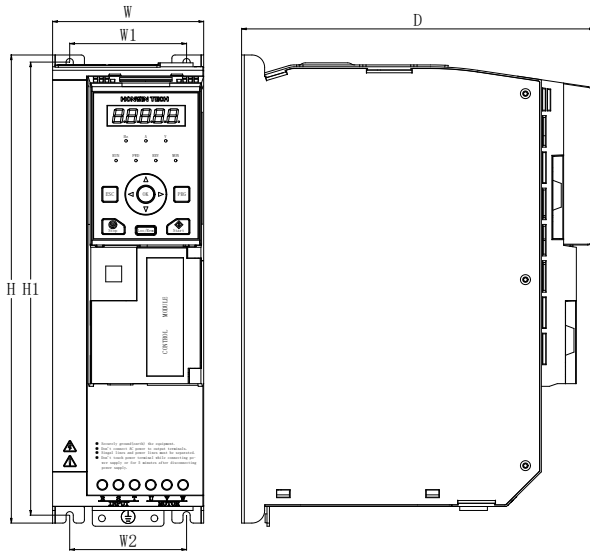
图 8-2 H100-4T7.5GB~H100-4T15GB 安装尺寸示意图
