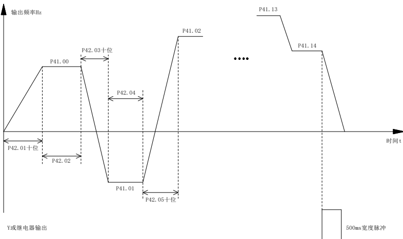
图 5-23 简易 PLC 运行示意图
