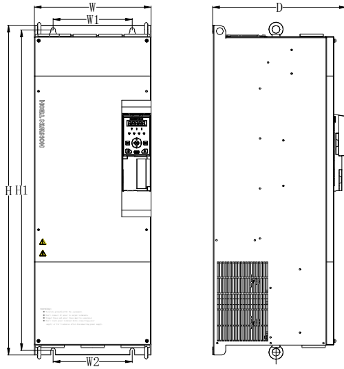
图 8-4 H100-4T37GB~H100-4T200G H100-4T315G~H100-4T450G 安装尺寸示意图
