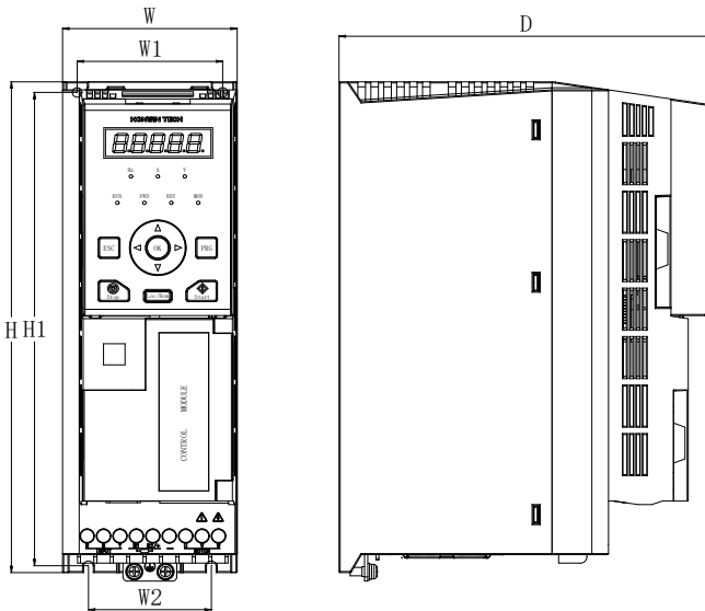
图 8-1 H100-4T5.5GB 及以下功率等级安装尺寸示意图
