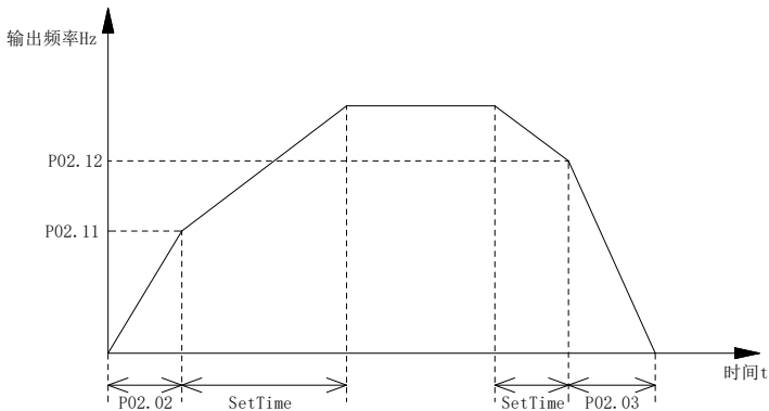
图 5-4 折线加减速时间切换示意图
